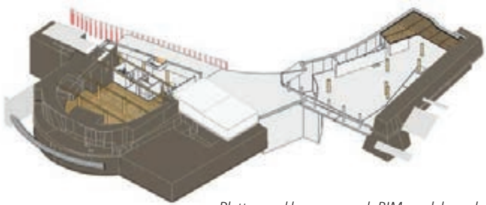
Plattegrond begane grond; BIM-model van de hoofdraagconstructie.
