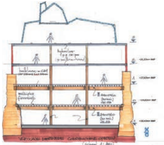
Verticale doorsnede; laagsgewijze stapeling van de verschillende constructiematerialen.
