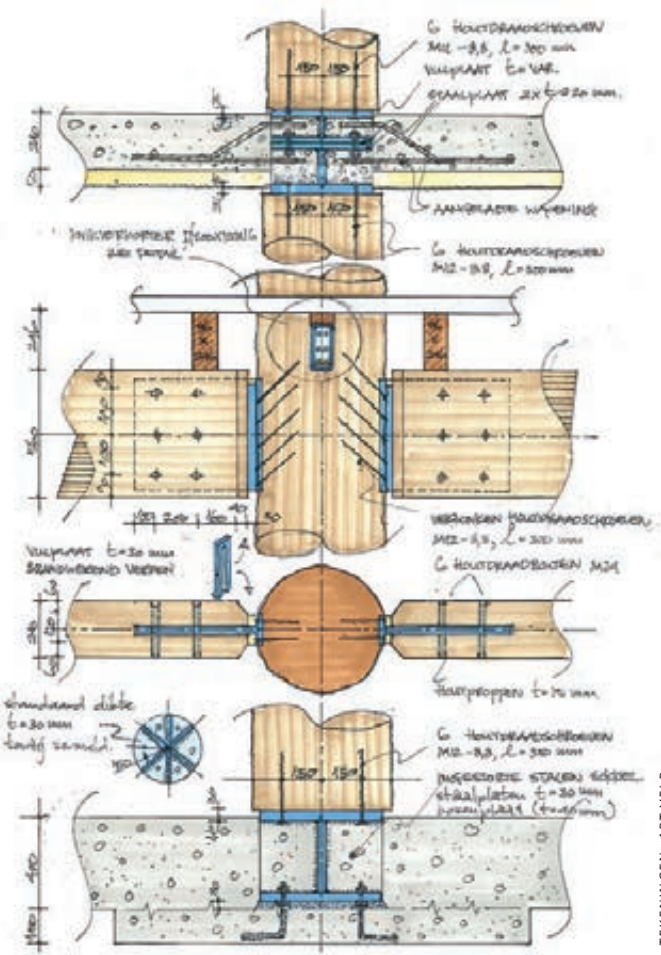
Aansluitdetails douglas stammen met de constructie.
