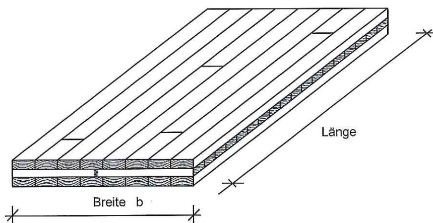
Bild A.2.2: Brettspertholzelement (hier: Beispiel mit drei Lagen)
