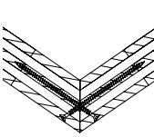
Schräger Stumpfstoß
