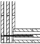
Einglassener Wandstoß
