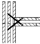
Einglassener Stoß, Vollgewindeschrauben schräg von innen
