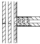
Stumpfstoß, einglassene Winkel und Kammnägel / Schrauben
