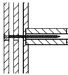
Einglassener Stoß, Vollgewindeschrauben senkrecht von außen
