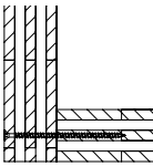
Rechtwinkliger Stumpfstoß
