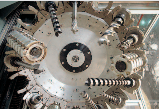
Werkzeugspindel CNC-Anlage
